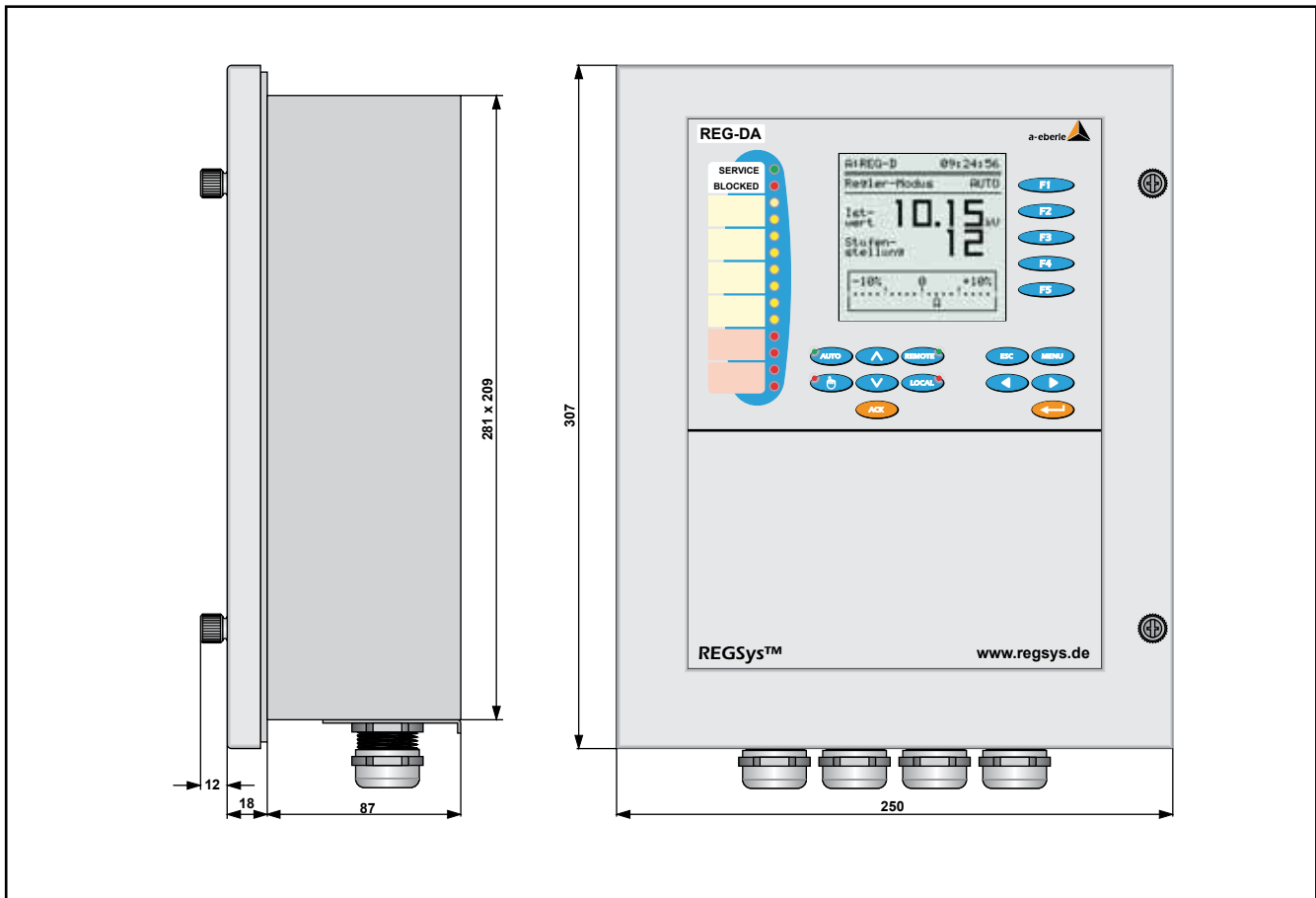
Mechanické rozměry
